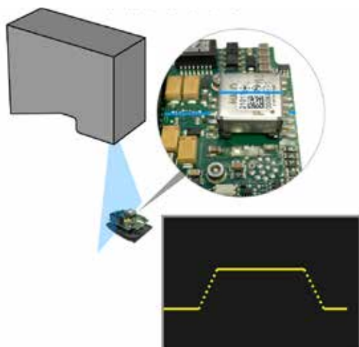
配备标准镜头的激光轮廓仪
